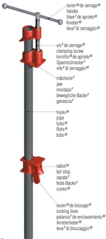
serre-joint M à tuyau M pipe clamp sargento M Rohrschraubstock M morsa F serratubi M
